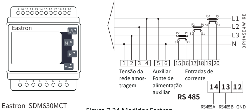
Figura 7.24 Medidor Eastron
