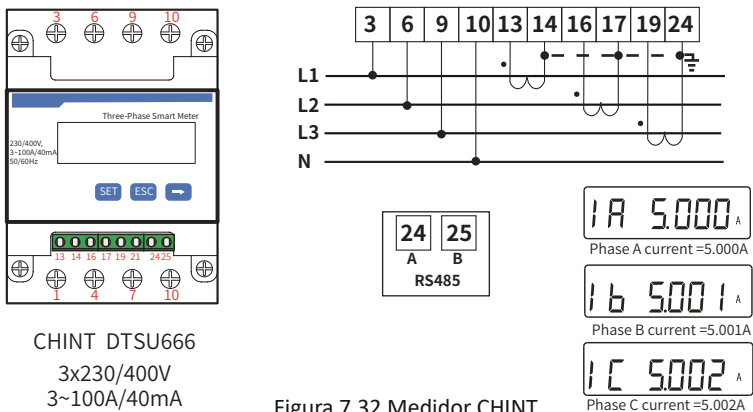
Figura 7.32 Medidor CHINT
