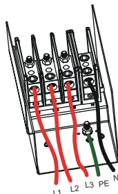
Figura 5.9 Condutor CA conectado ao terminal
