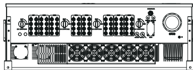
Figura 1.2 Vista inferior
